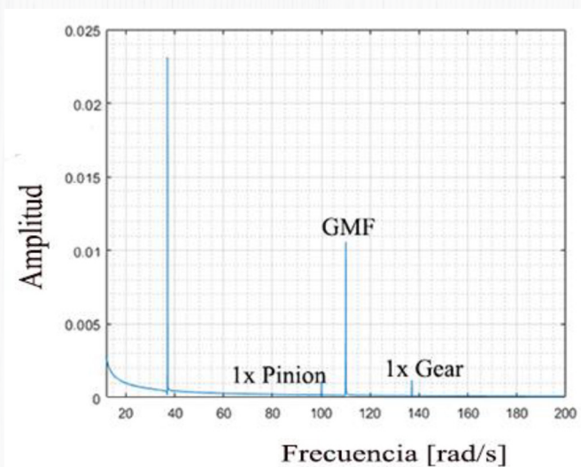
Figura 8. Espectro en frecuencia con la falla sobrecarga de los dientes de engrane
