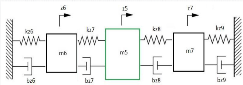
Figura 1. Representación grados de libertad axiales
